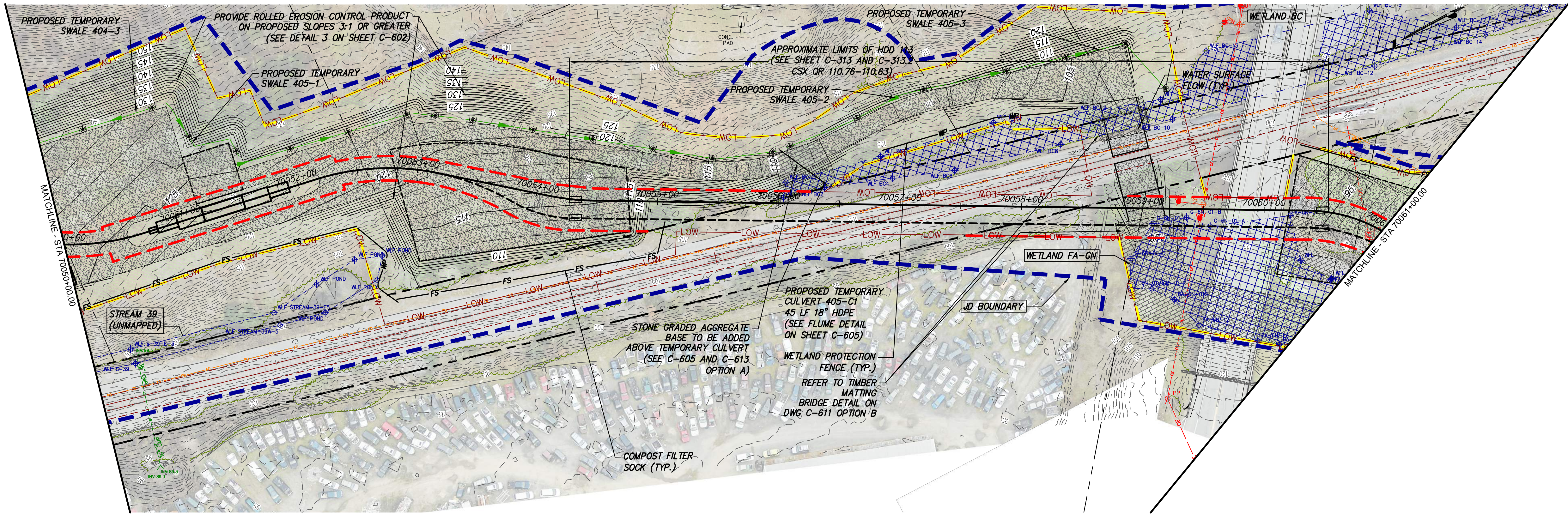
STA. 70050+00.00 TO STA. 70061+00.00 PLAN VIEW SCALE: 1" = 50'
