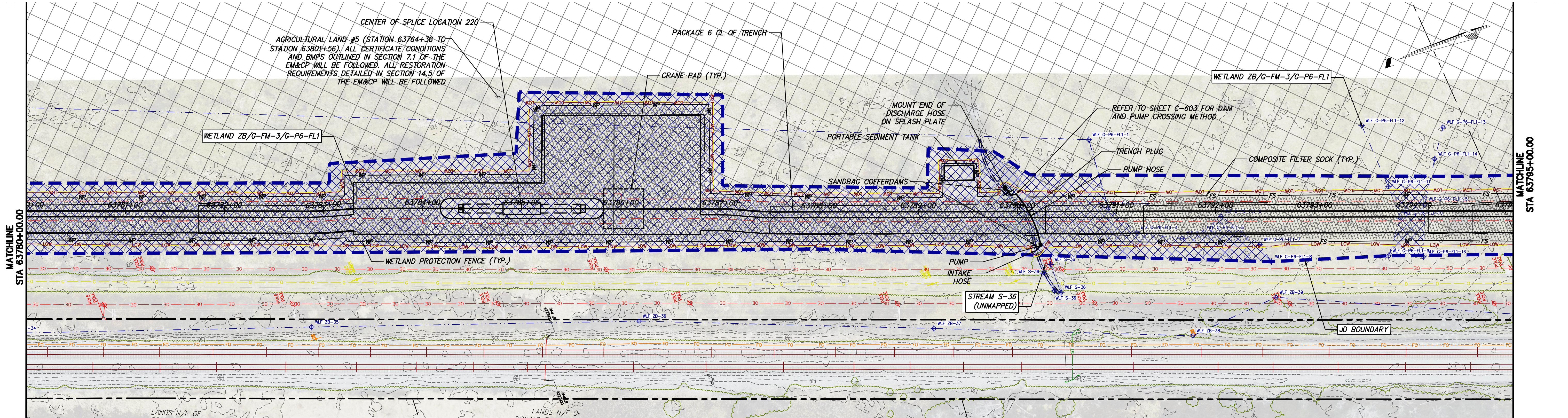
STA. 63780+00 TO STA. 63795+00 PLAN VIEW SCALE: 1" = 50'
