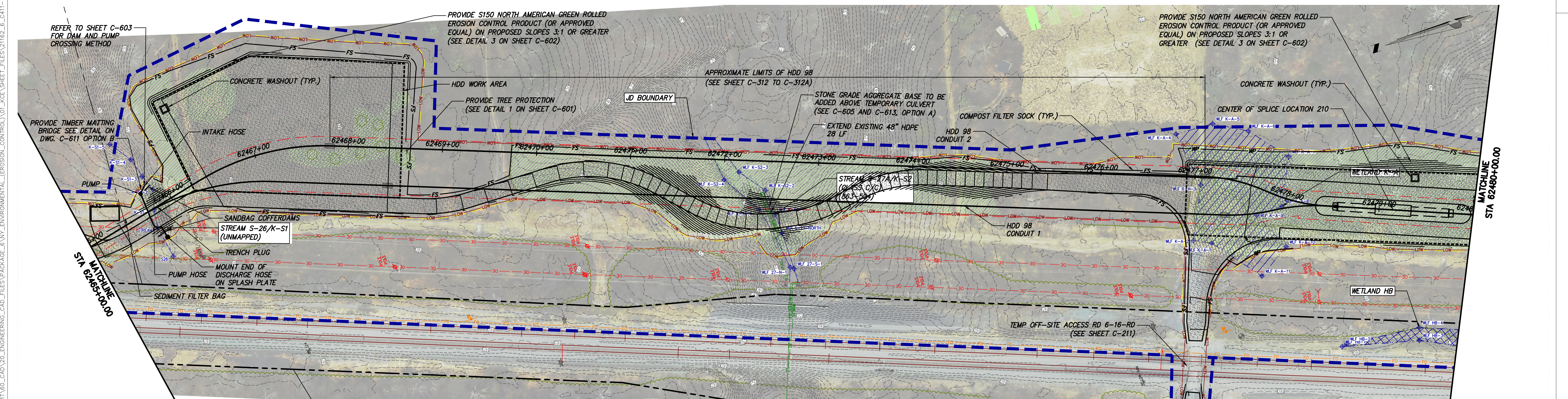
STA. 62465+00 TO STA. 62480+00 PLAN VIEW SCALE: 1" = 50'
