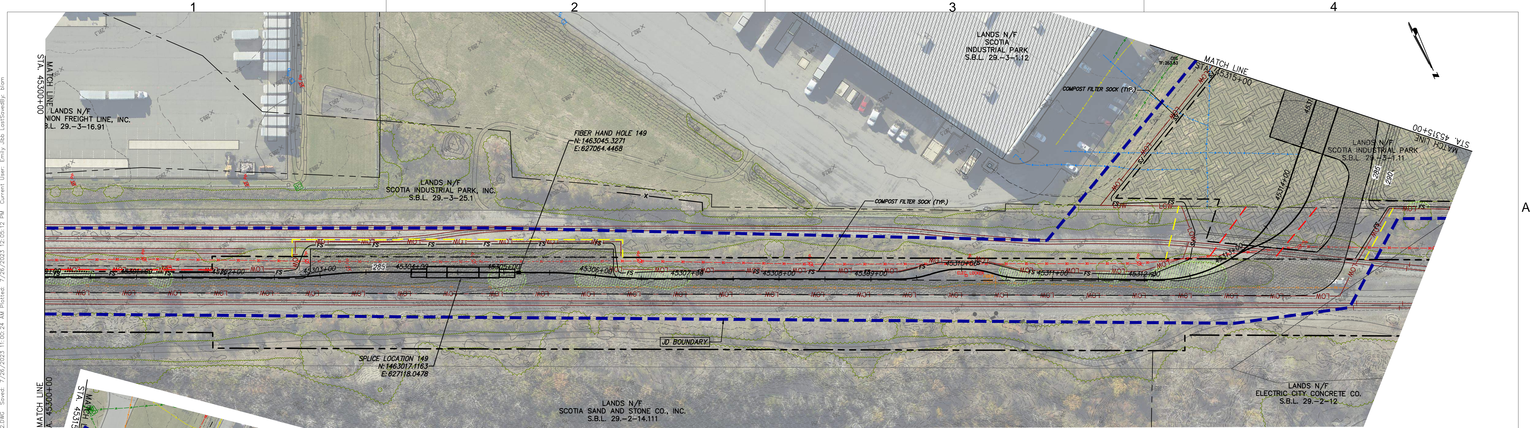
STA. 45300+00 TO STA. 45315+00 PLAN VIEW SCALE: 1" = 50'
