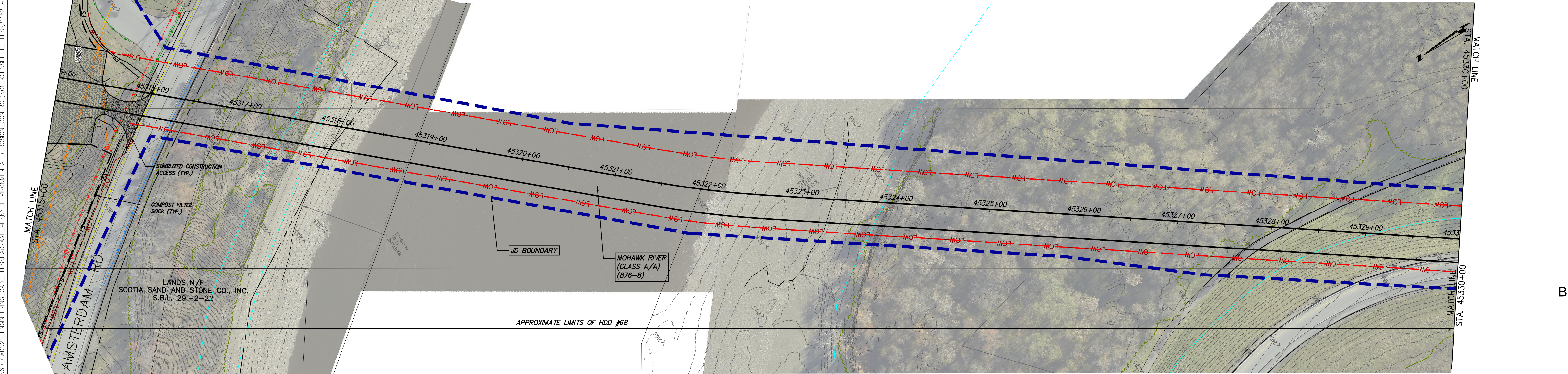
STA. 45315+00 TO STA. 45330+00 PLAN VIEW SCALE: 1" = 50'
