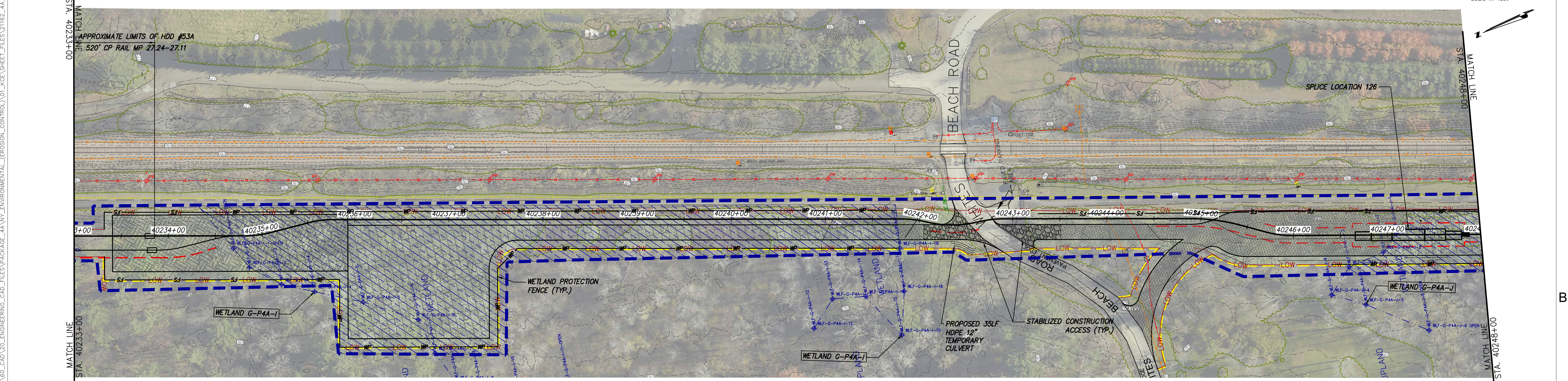
STA. 40233+00 TO STA. 40248+00 PLAN VIEW SCALE: 1" = 50'
