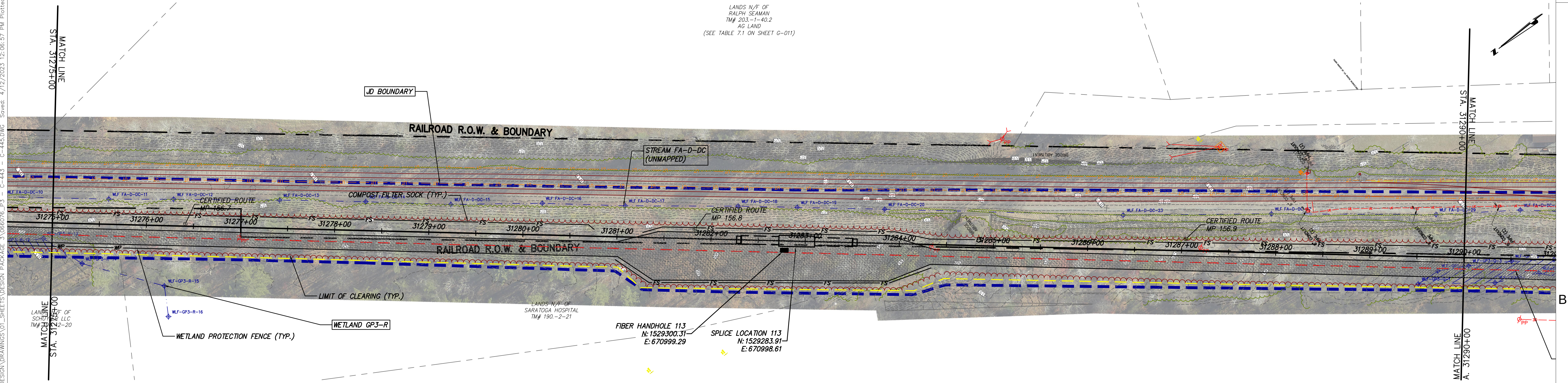
STA. 31275+00 TO STA. 31290+00 PLAN VIEW SCALE: H:1" = 50' V:1" = 10'
