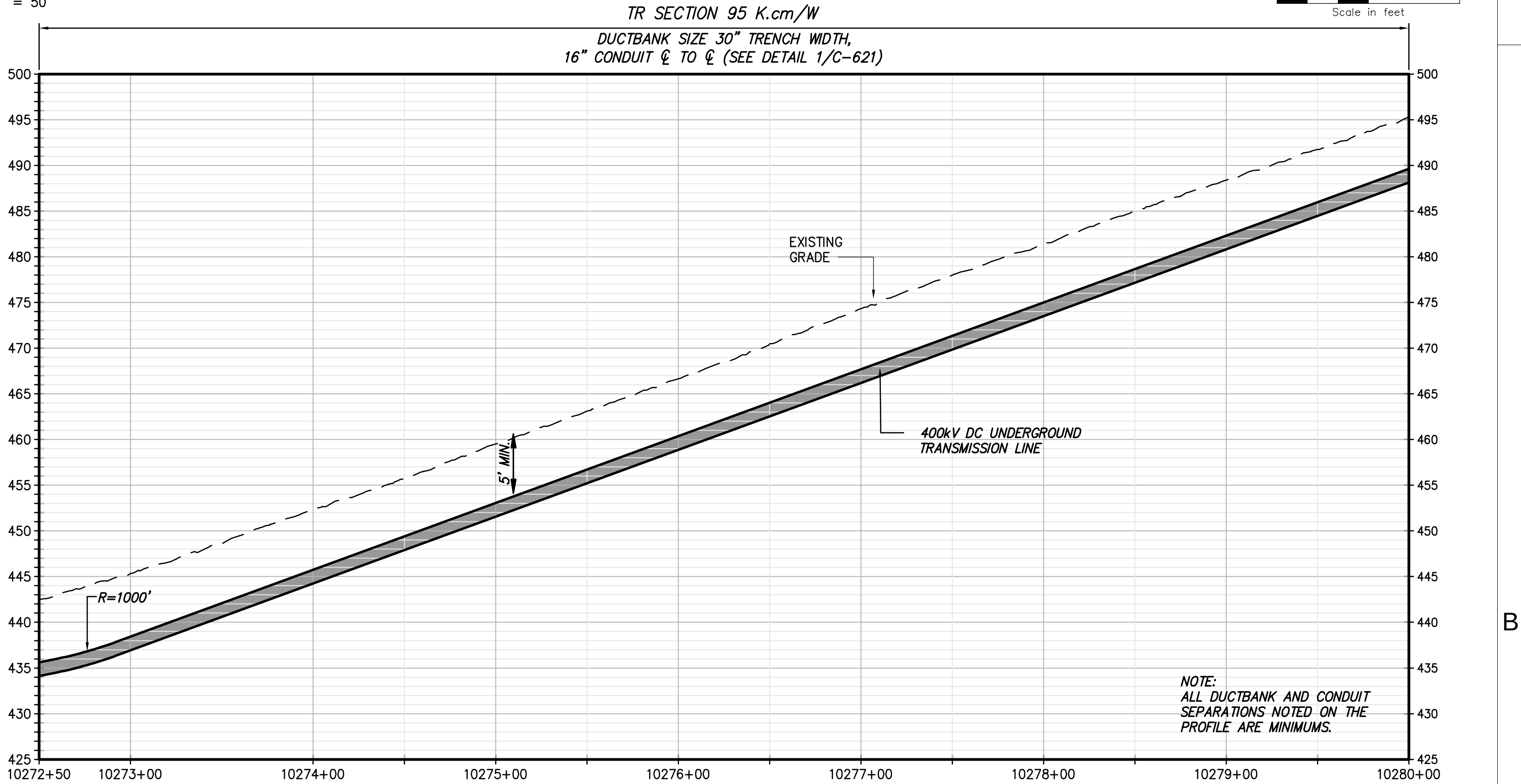
STA. 10272+50 TO STA. 10280+00 PROFILE VIEW SCALE: H:1" = 50' V:1" = 10'
