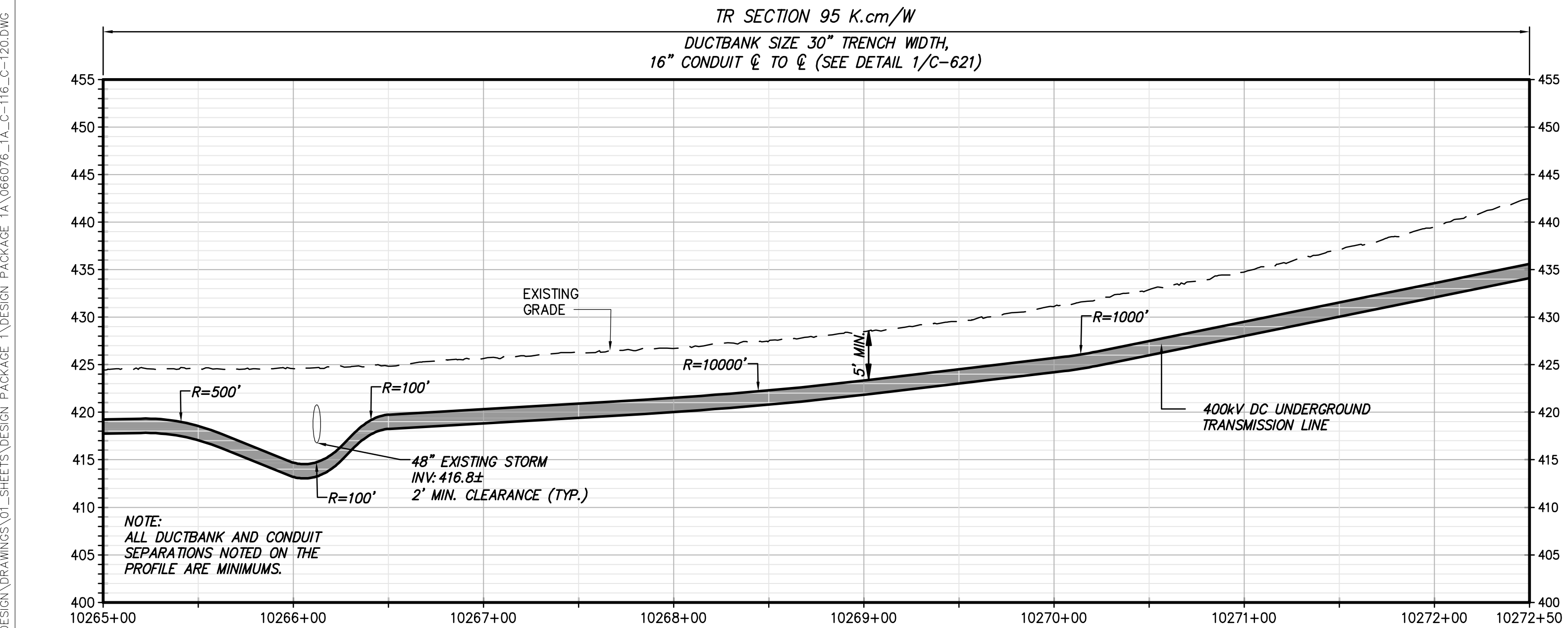
STA. 10265+00 TO STA. 10272+50 PROFILE VIEW SCALE: H:1" = 50' V:1" = 10'
