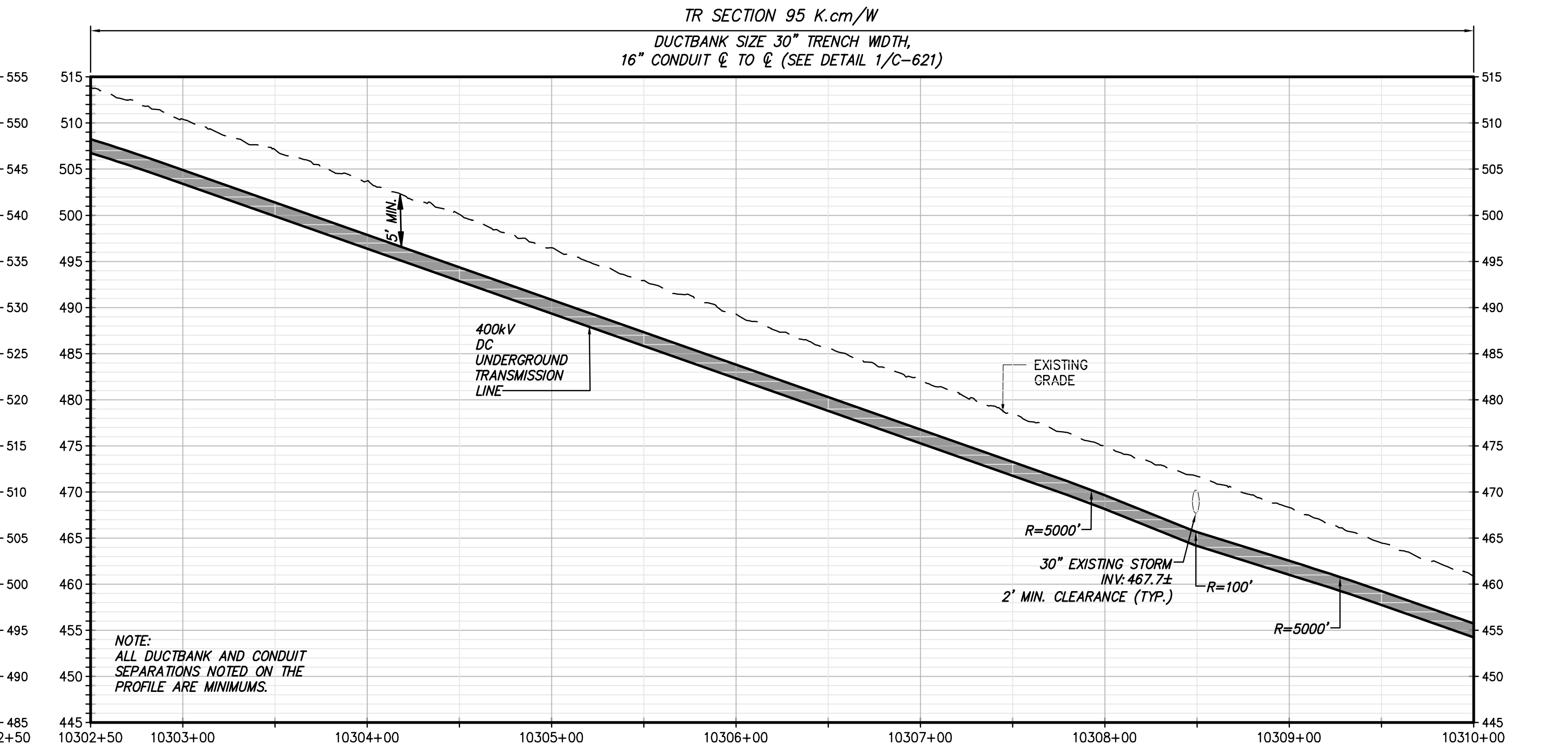
STA. 10302+50 TO STA. 10310+00 PROFILE VIEW SCALE: H: 1" = 50' V: 1" = 10'
