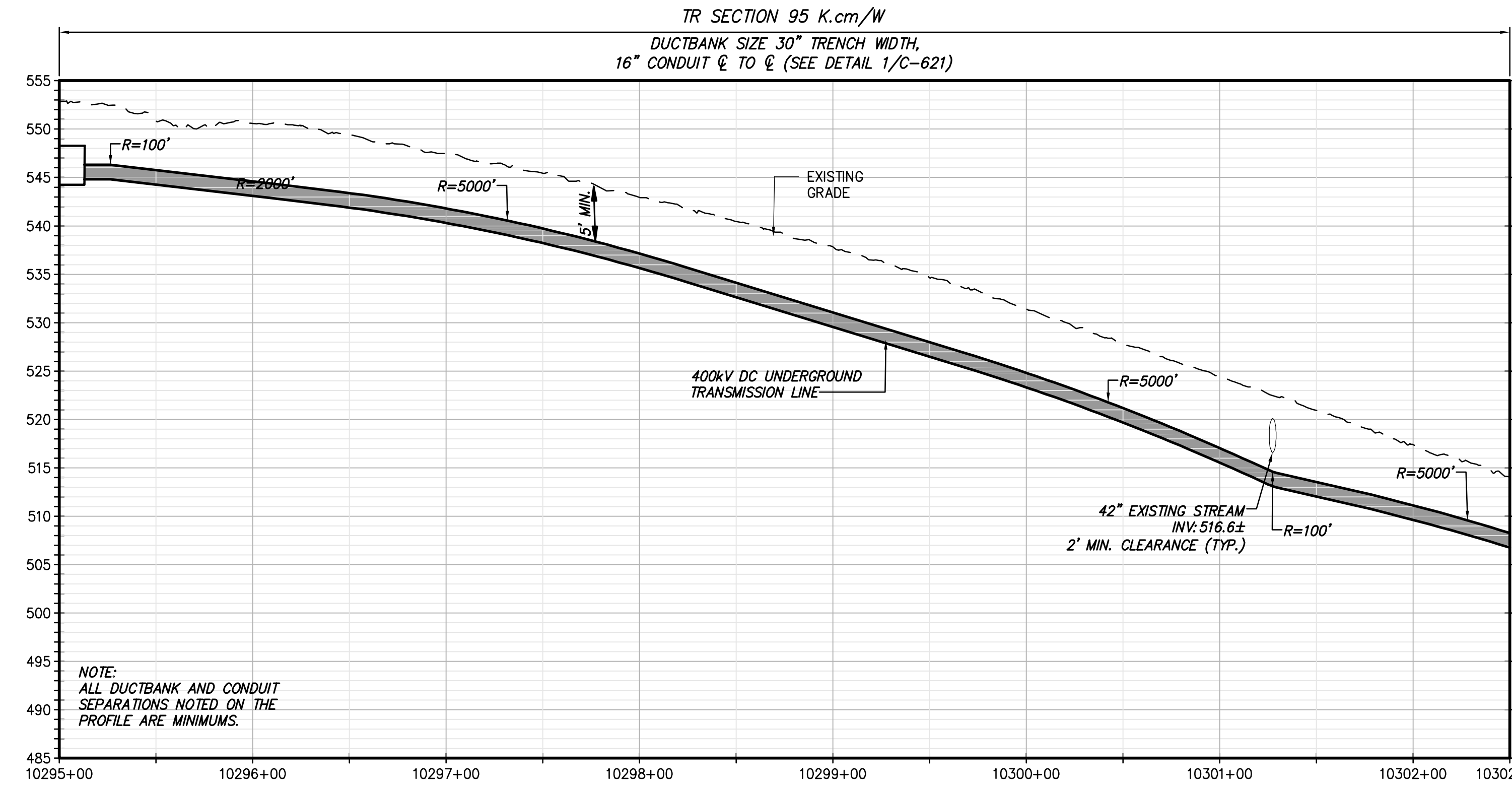
STA. 10295+00 TO STA. 10302+50 PROFILE VIEW SCALE: H: 1" = 50' V: 1" = 10'
