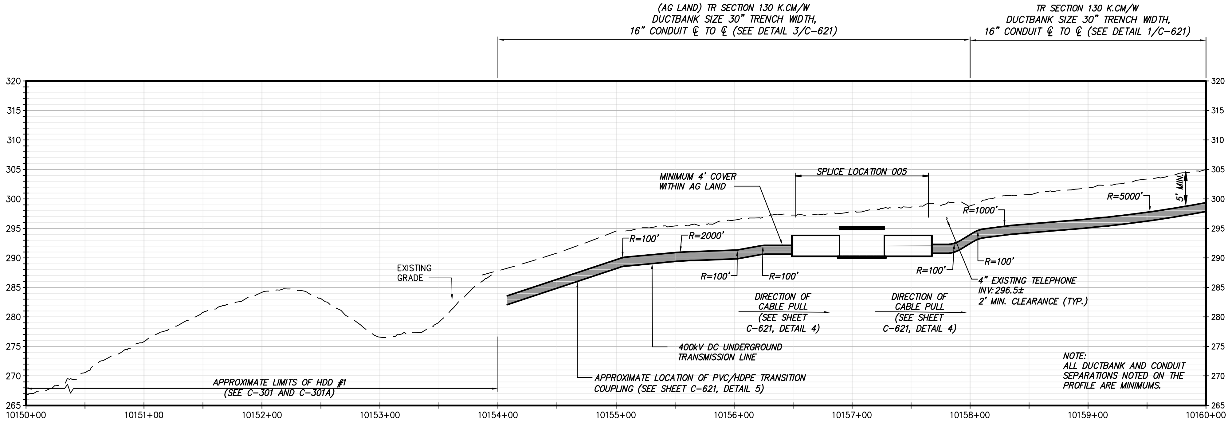
STA. 10150+00 TO STA. 10160+00 PROFILE VIEW SCALE: H: 1" = 50' V: 1" = 10'
