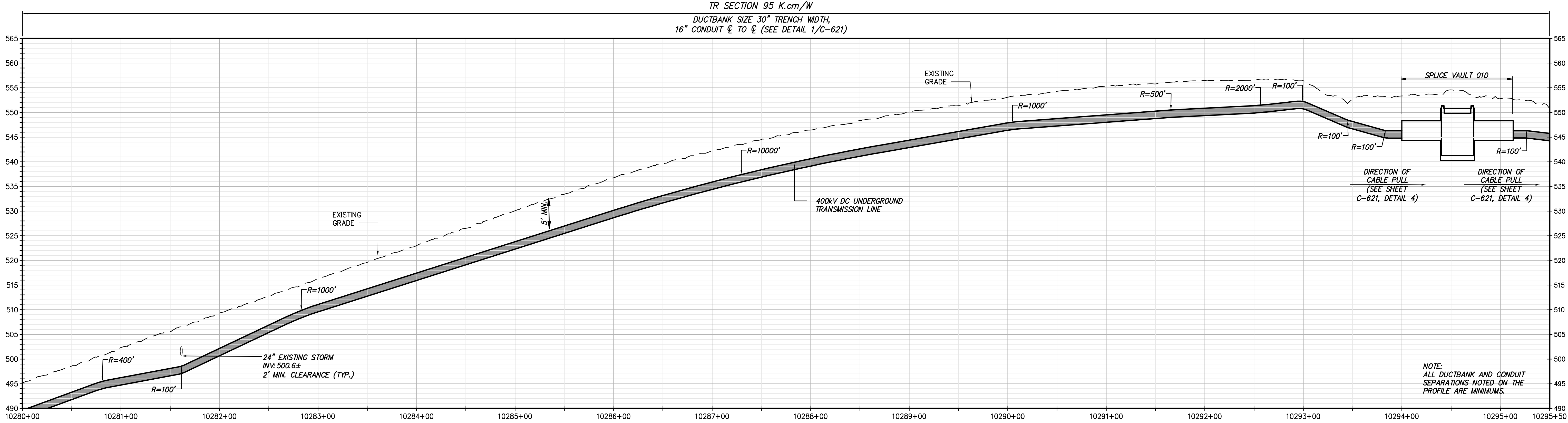
STA. 10280+00 TO STA. 10295+00 PROFILE VIEW SCALE: H:1" = 50' V:1" = 10'
