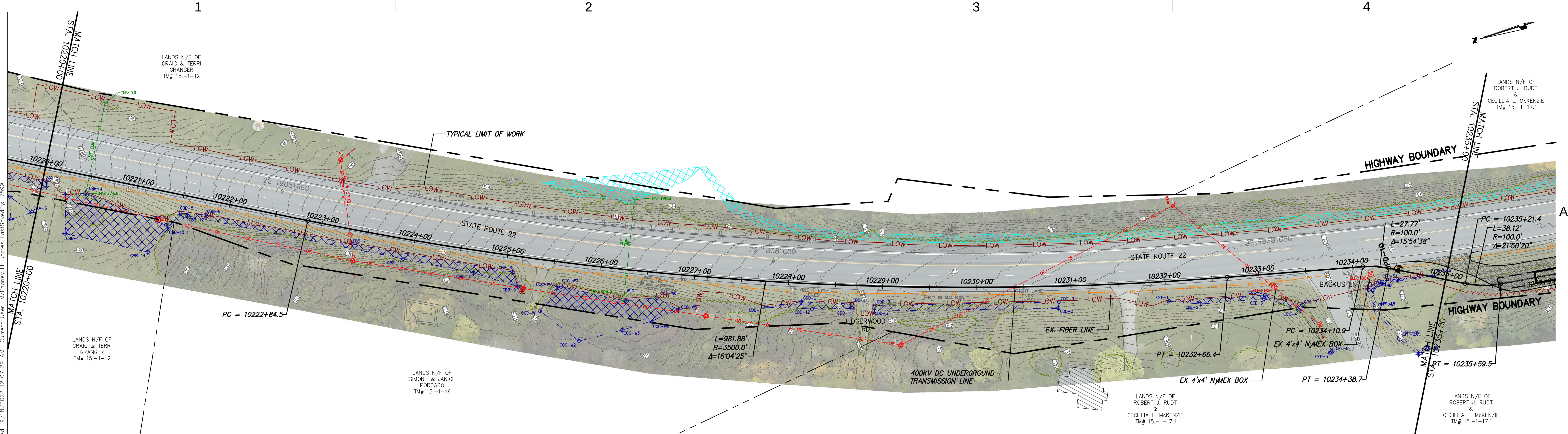
STA. 10220+00 TO STA. 10235+00 PLAN VIEW SCALE: 1" = 50'
