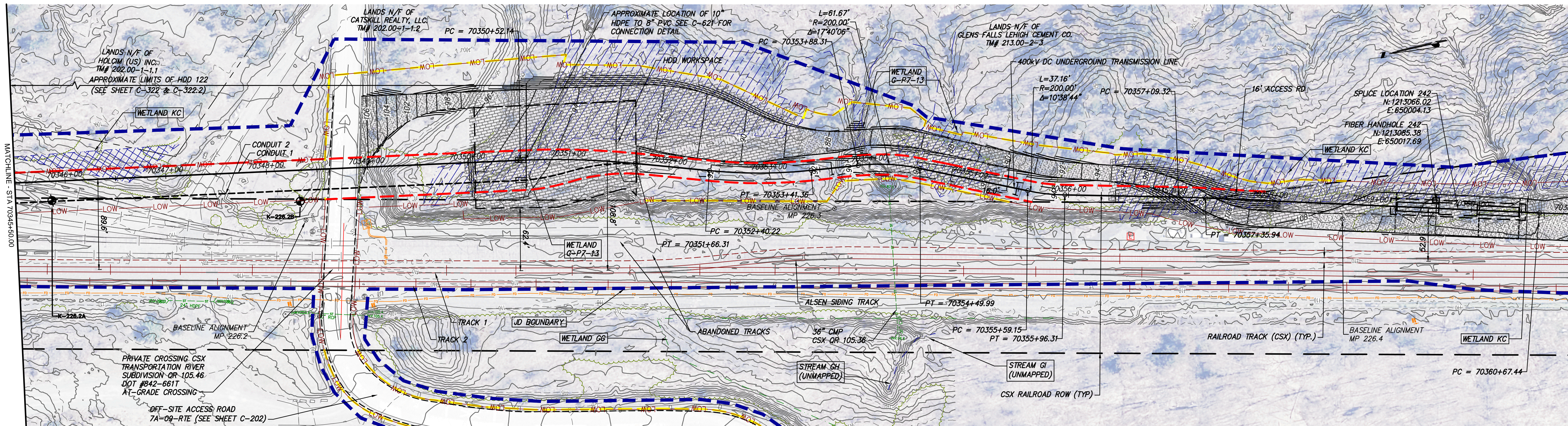
STA. 70345+50.00 TO STA. 70361+00.00 PLAN VIEW SCALE: 1" = 50'
