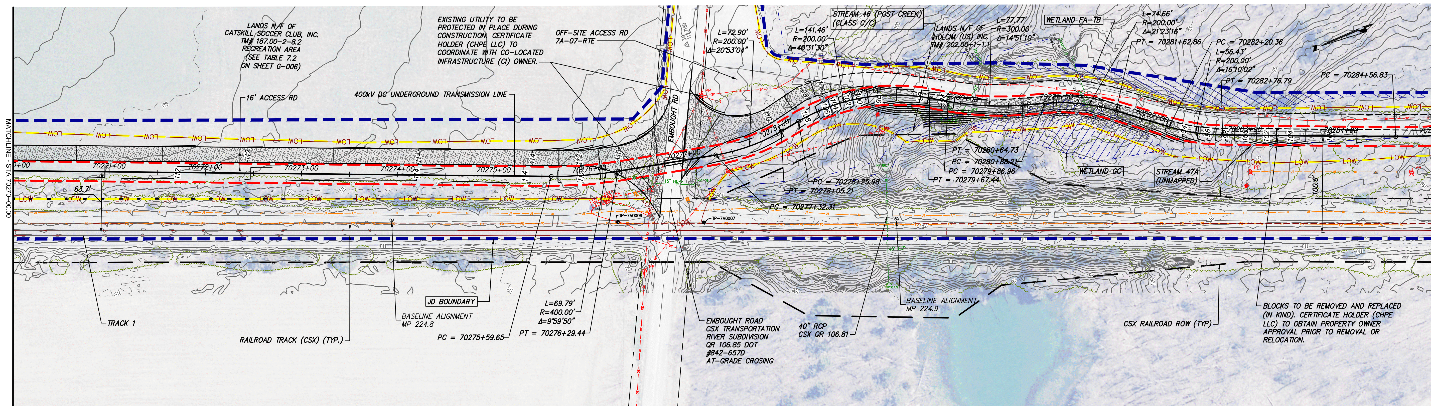
STA. 70270+00.00 TO STA. 70285+00.00 PLAN VIEW SCALE: 1" = 50'
