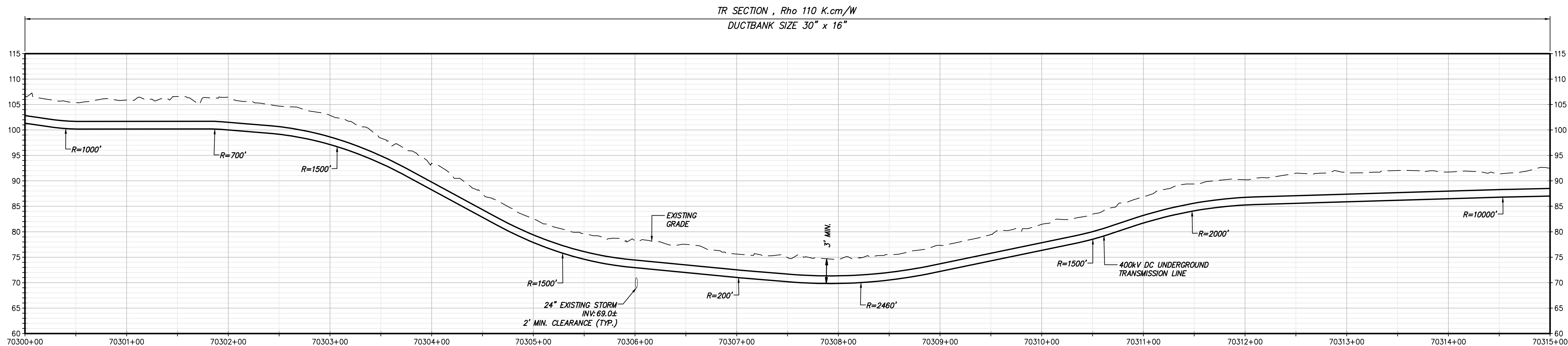
STA. 70300+00 TO STA. 70315+00 PROFILE VIEW SCALE: H:1" = 50' V:1" = 10'
