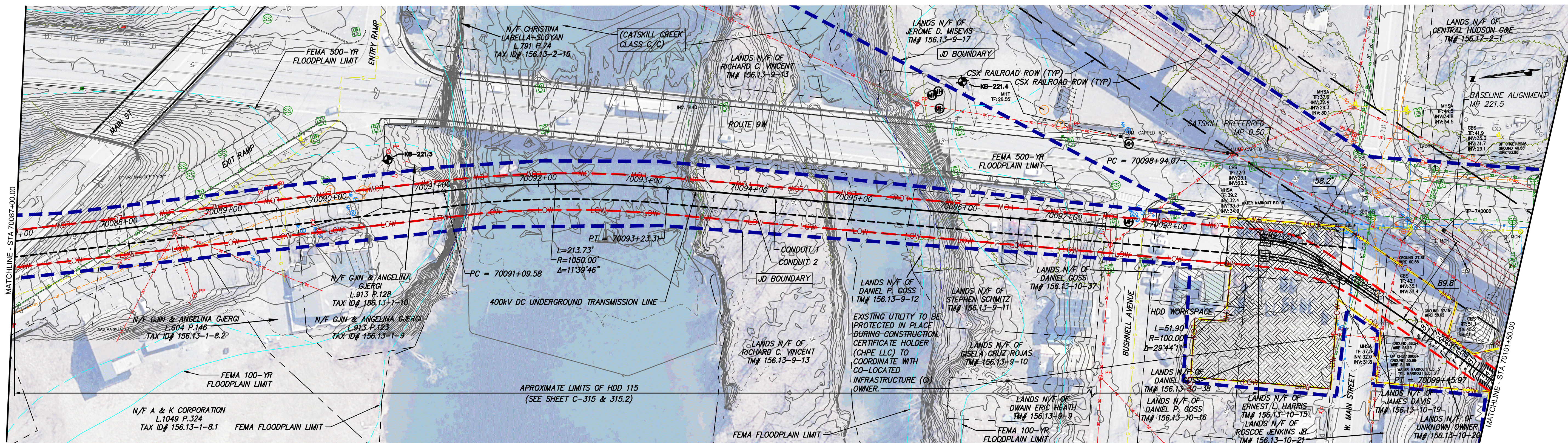
STA. 70087+00.00 TO STA. 70101+50.00 PLAN VIEW SCALE: 1" = 50'
