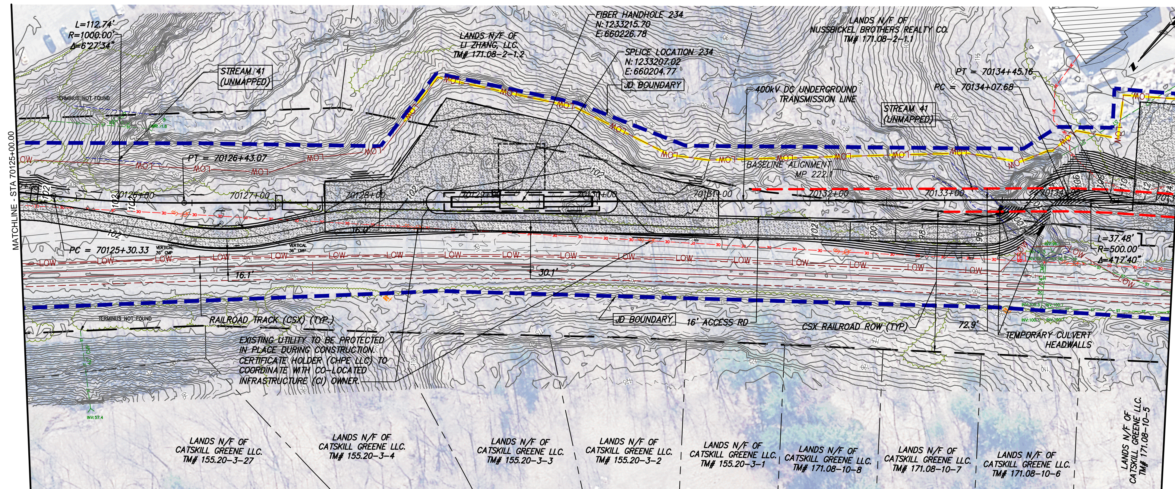
STA. 70125+00.00 TO STA. 70135+00.00 PLAN VIEW SCALE: 1" = 50'
