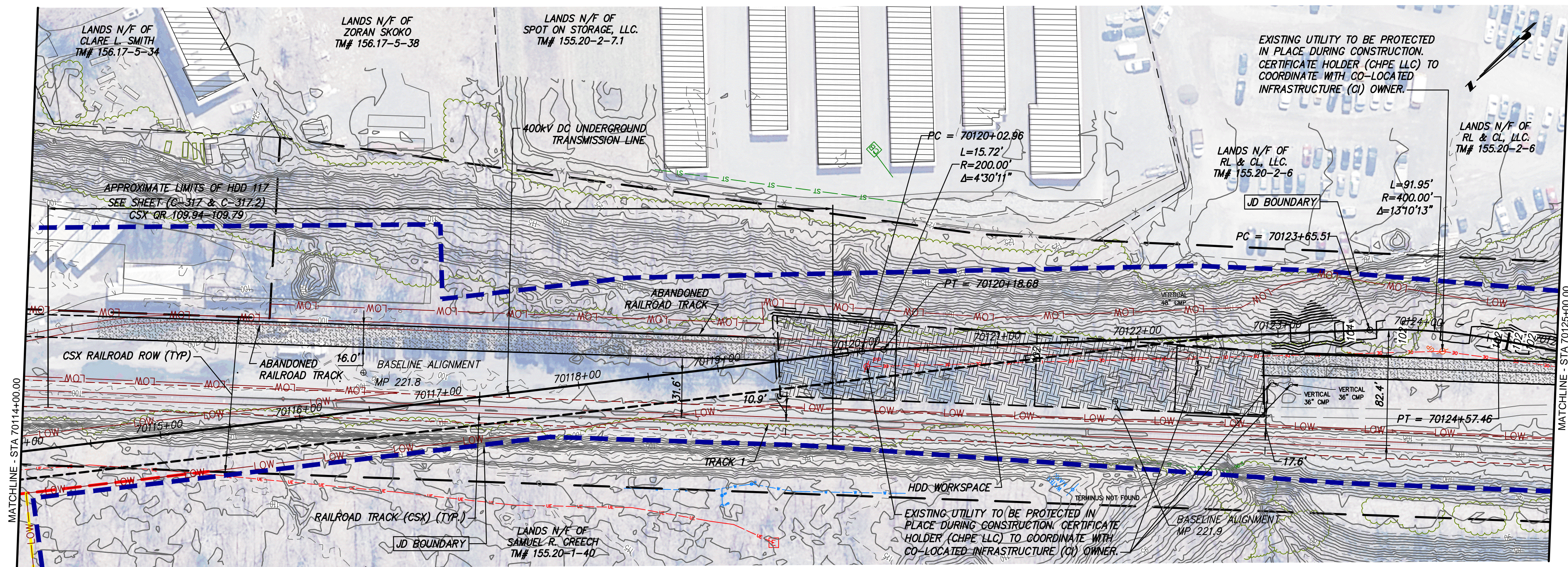
STA. 70114+00.00 TO STA. 70125+00.00 PLAN VIEW SCALE: 1" = 50'
