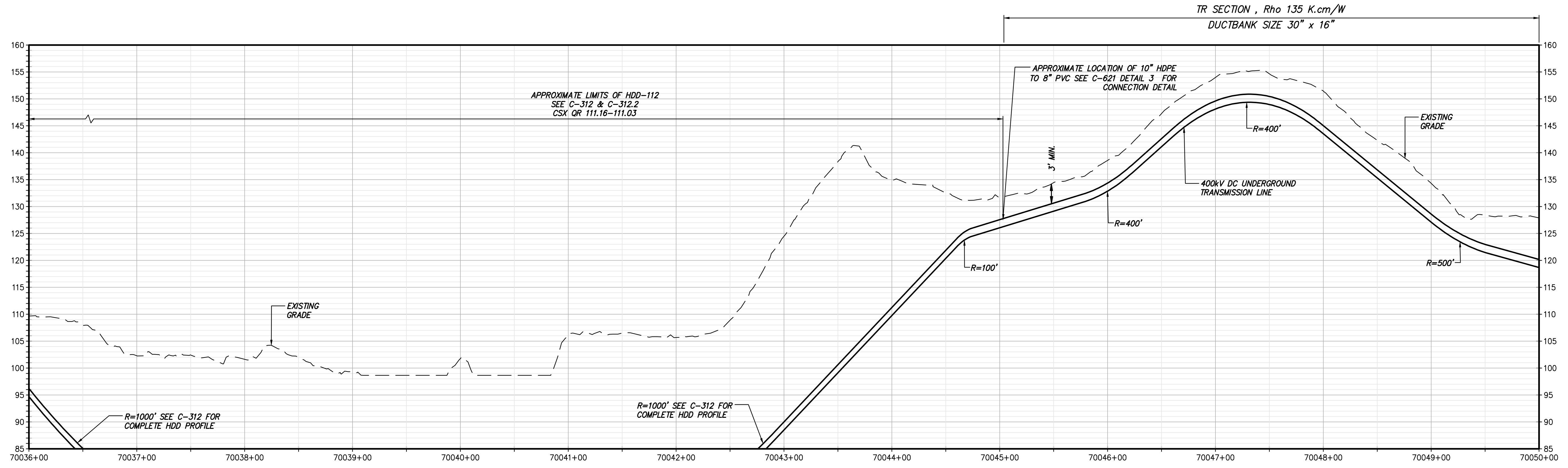
STA. 70036+00 TO STA. 70050+00 PROFILE VIEW SCALE: H: 1" = 50' V: 1" = 10'
