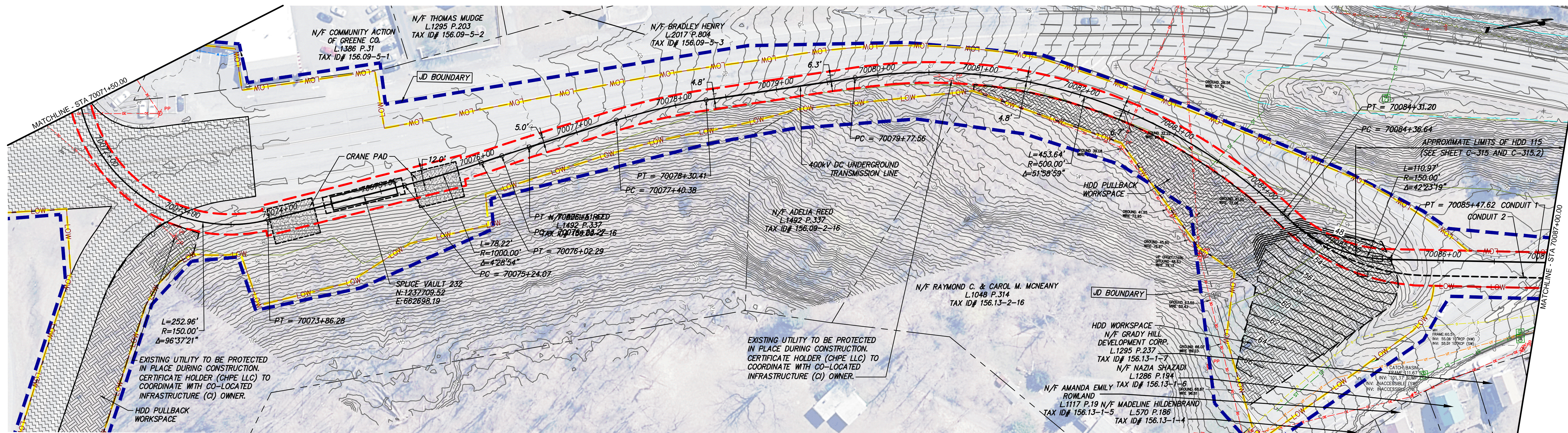
STA. 70071+50.00 TO STA. 70087+00.00 PLAN VIEW SCALE: 1" = 50'
