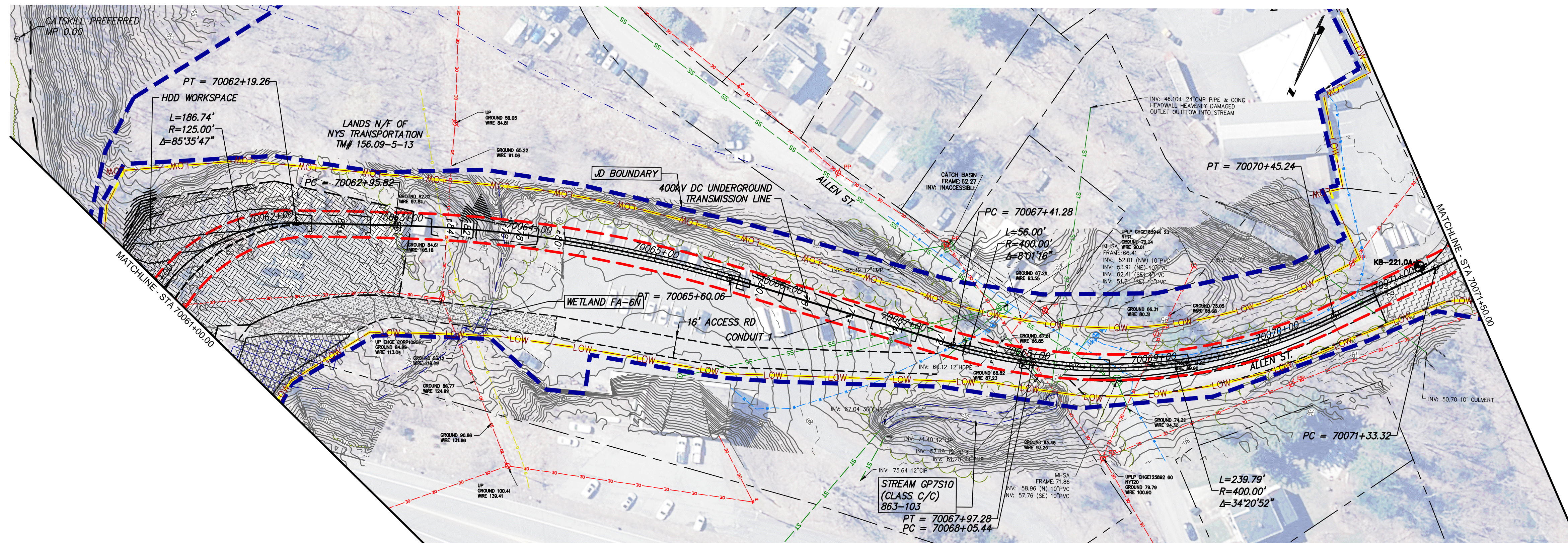
STA. 70061+00.00 TO STA. 70071+50.00 PLAN VIEW SCALE: 1" = 50'
