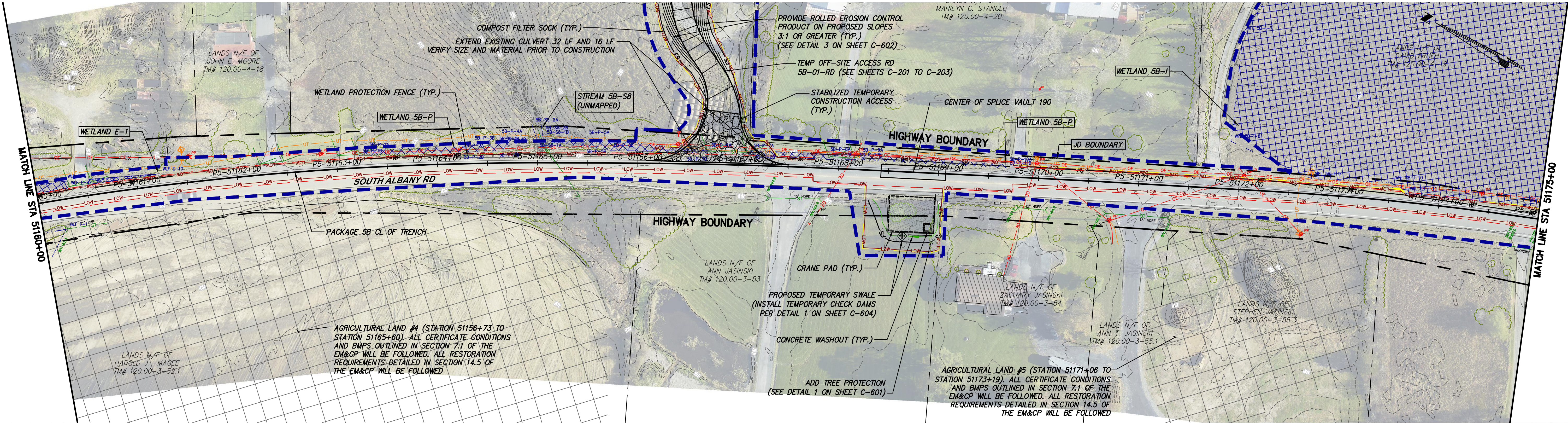
STA. 51160+00 TO STA. 51175+00 PLAN VIEW SCALE: 1" = 50'
