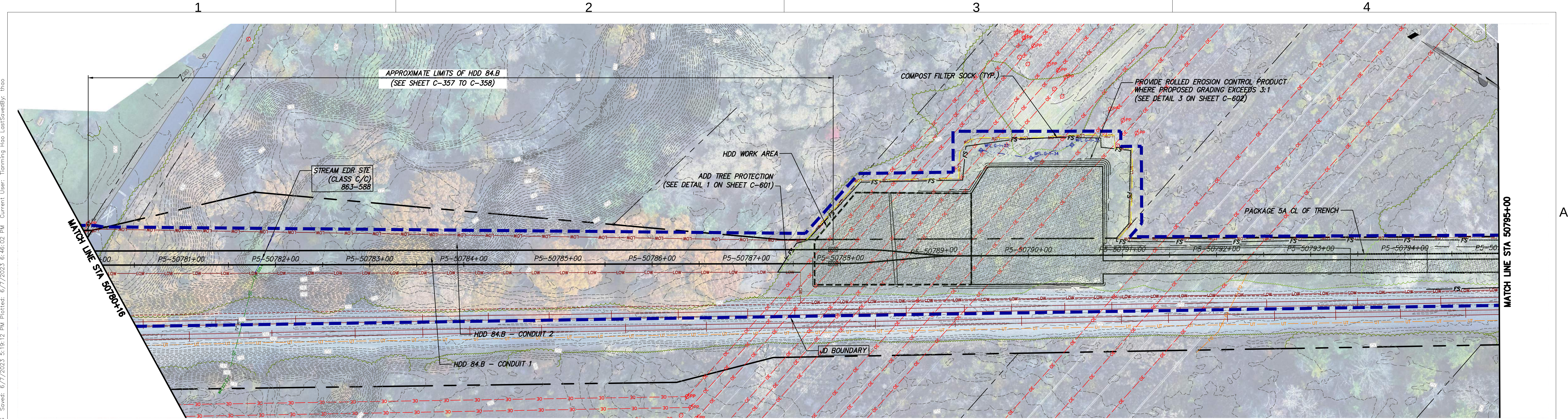
STA. 50780+00 TO STA. 50795+00 PLAN VIEW SCALE: 1" = 50'
