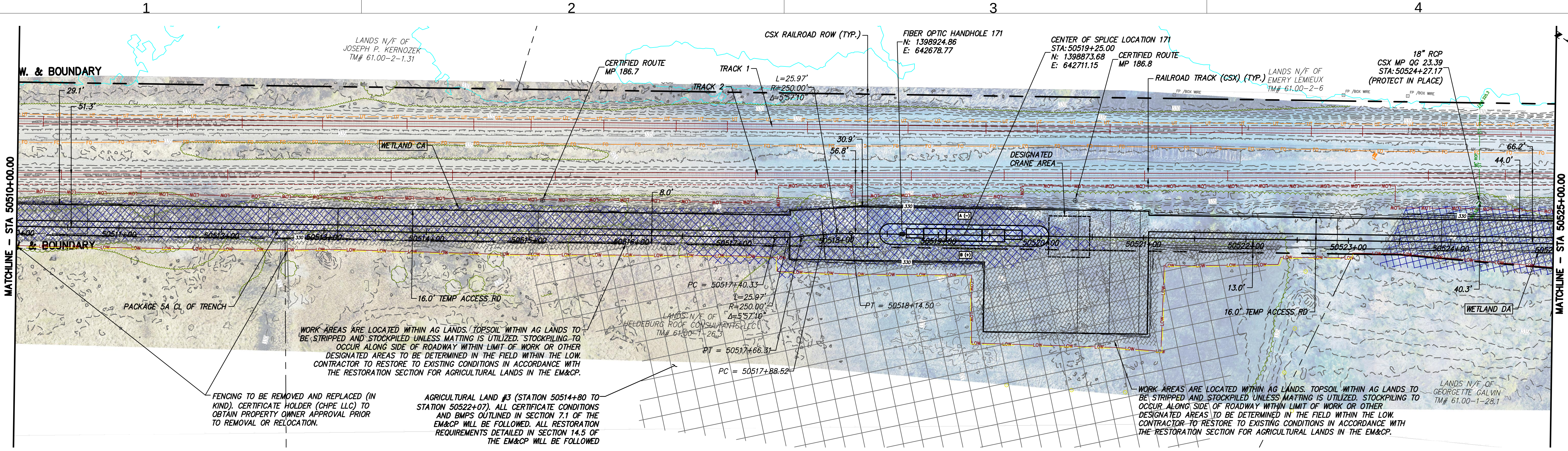
STA. 50510+00.00 TO STA. 50525+00.00 PLAN VIEW SCALE: 1" = 50'
