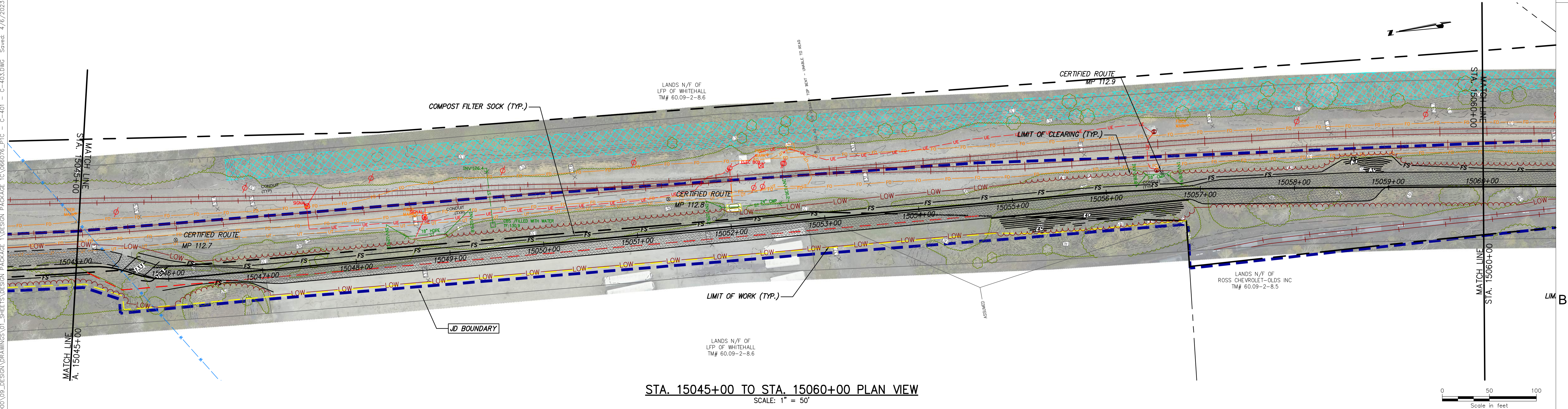
STA. 15030+00 TO STA. 15045+00 PLAN VIEW SCALE: 1" = 50'
