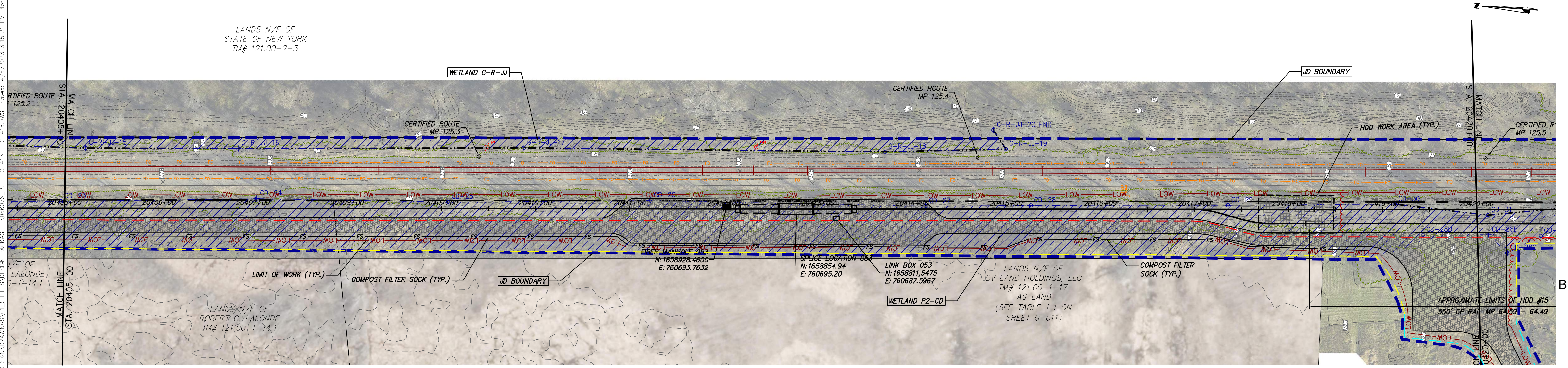
STA. 20405+00 TO STA. 20420+00 PLAN VIEW SCALE: 1" = 50'
