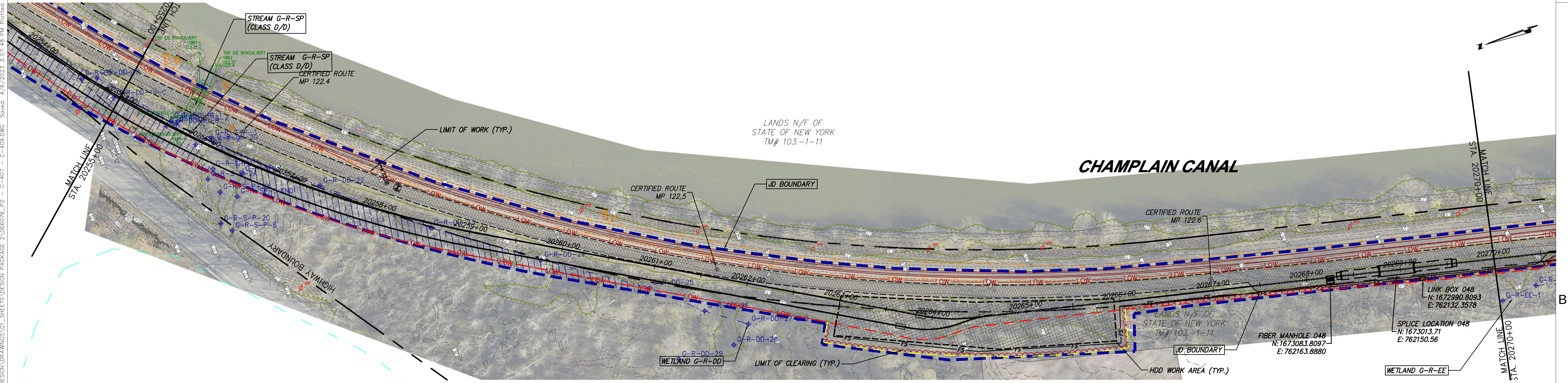
STA. 20255+00 TO STA. 20270+00 PLAN VIEW SCALE: 1" = 50'
