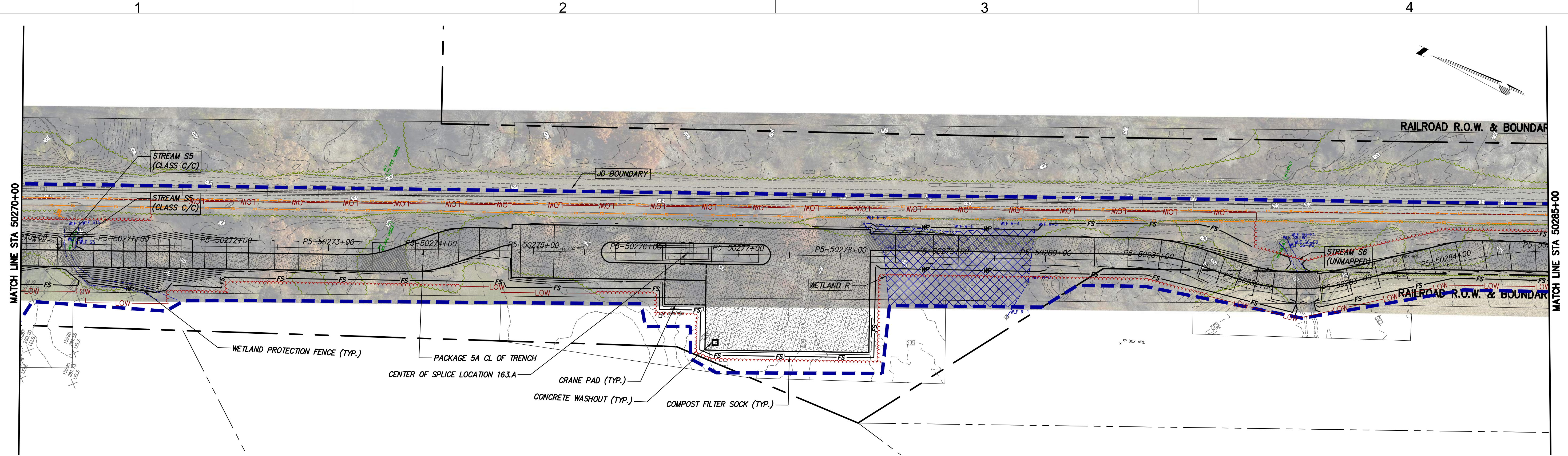
STA. 50270+00 TO STA. 50285+00 PLAN VIEW SCALE: 1" = 50'
