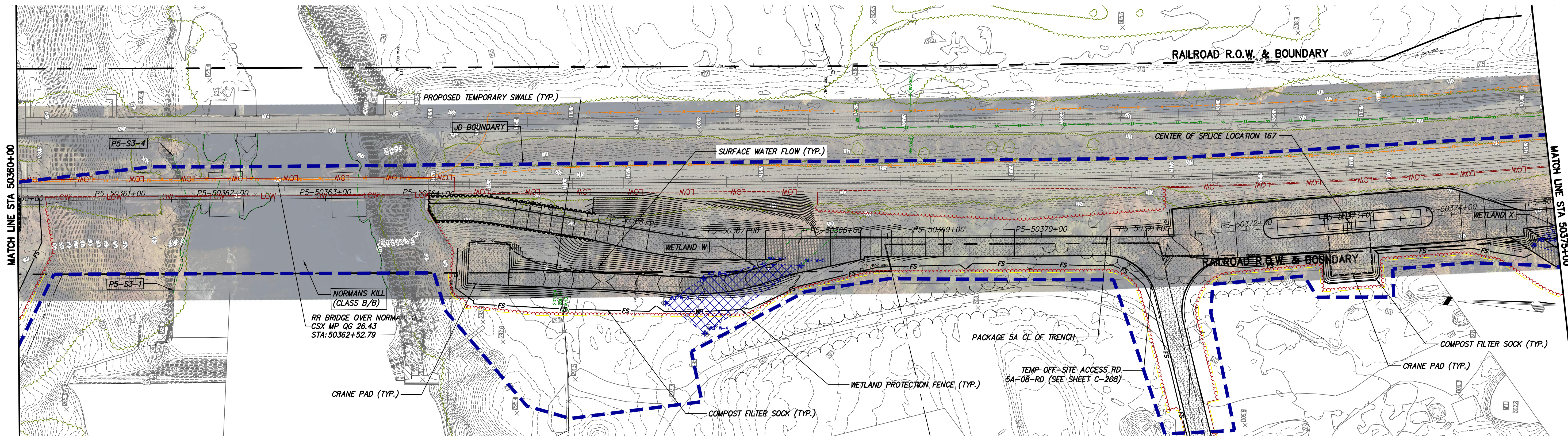
STA. 50360+00 TO STA. 50375+00 PLAN VIEW SCALE: 1" = 50'
