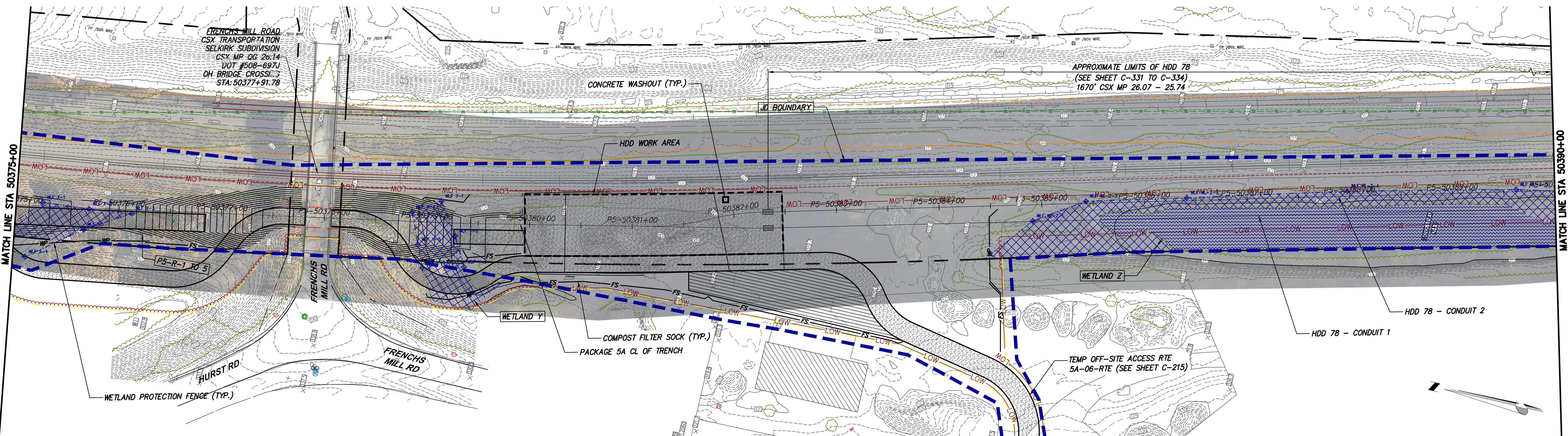
STA. 50375+00 TO STA. 50390+00 PLAN VIEW SCALE: 1" = 50'
