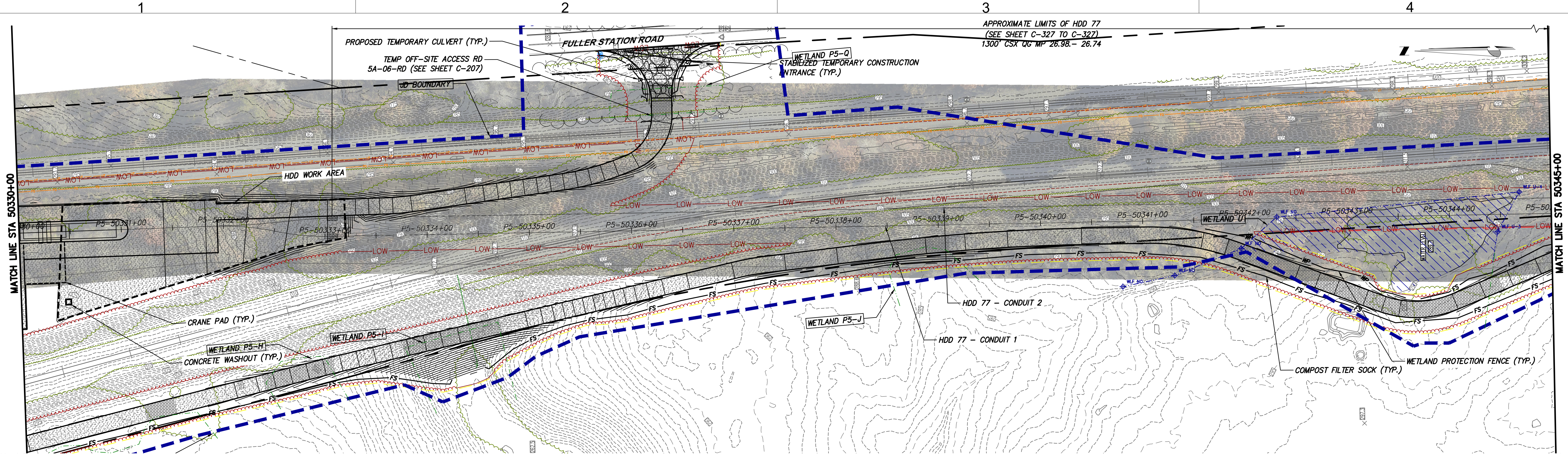
STA. 50330+00 TO STA. 50345+00 PLAN VIEW SCALE: 1" = 50'
