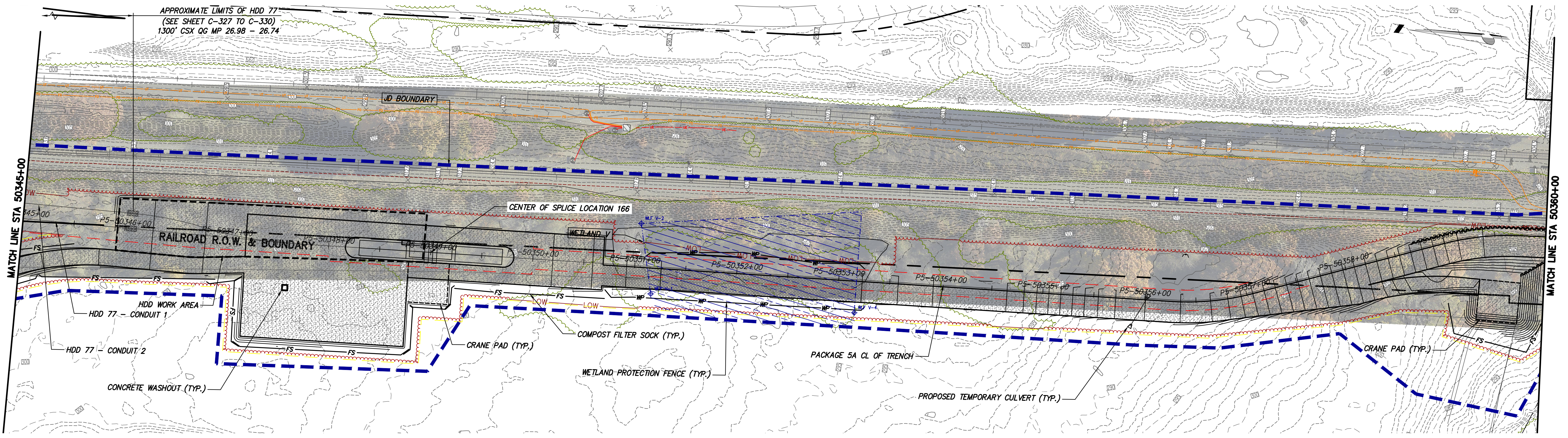
STA. 50345+00 TO STA. 50360+00 PLAN VIEW SCALE: 1" = 50'
