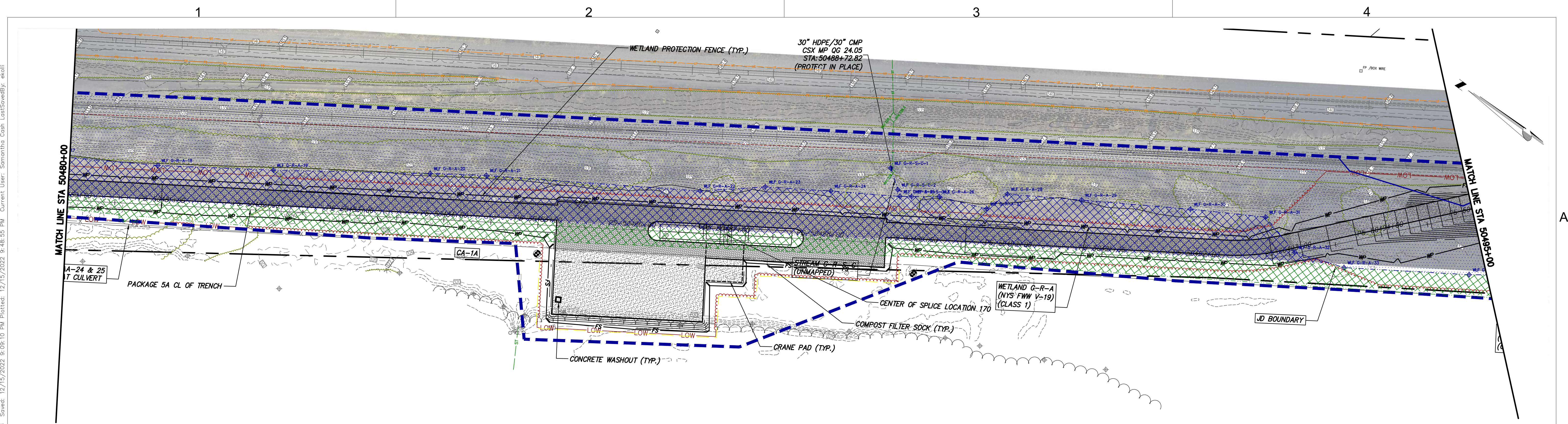
STA. 50480+00 TO STA. 50495+00 PLAN VIEW SCALE: 1" = 50'
