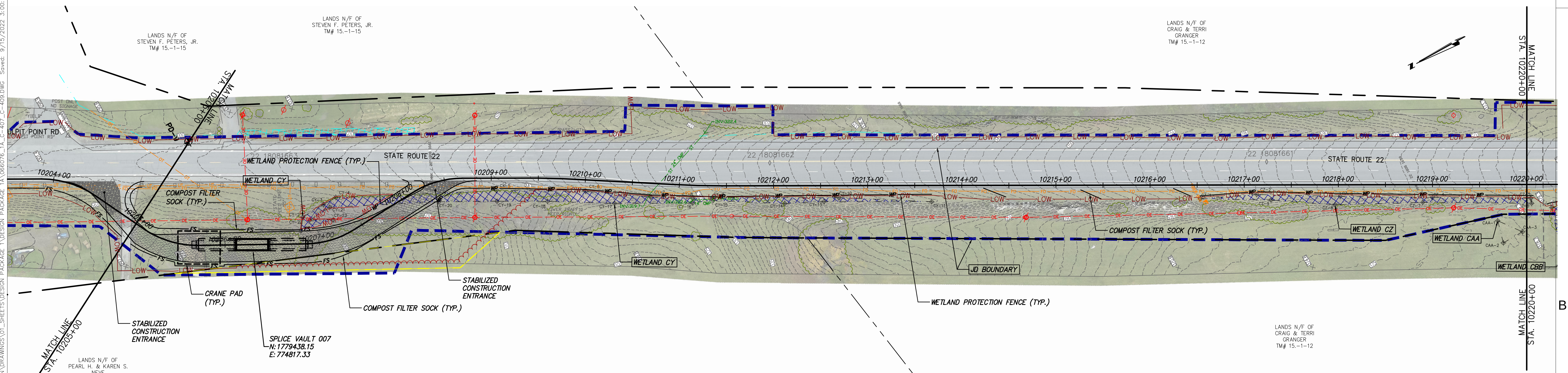
STA. 10205+00 TO STA. 10220+00 PLAN VIEW SCALE: 1" = 50'
