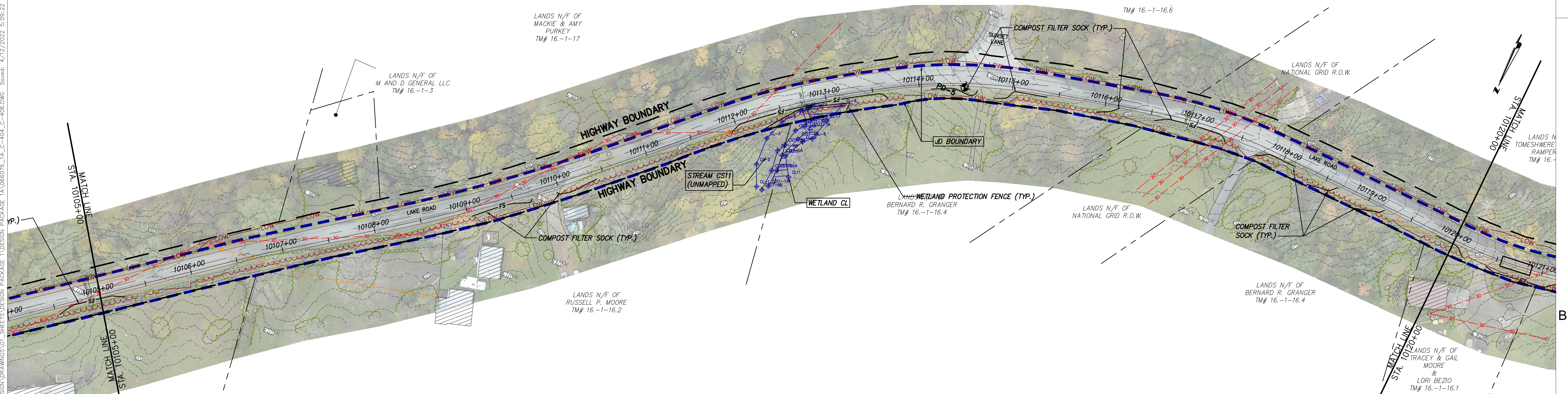
STA. 10105+00 TO STA. 10120+00 PLAN VIEW SCALE: 1" = 50'
