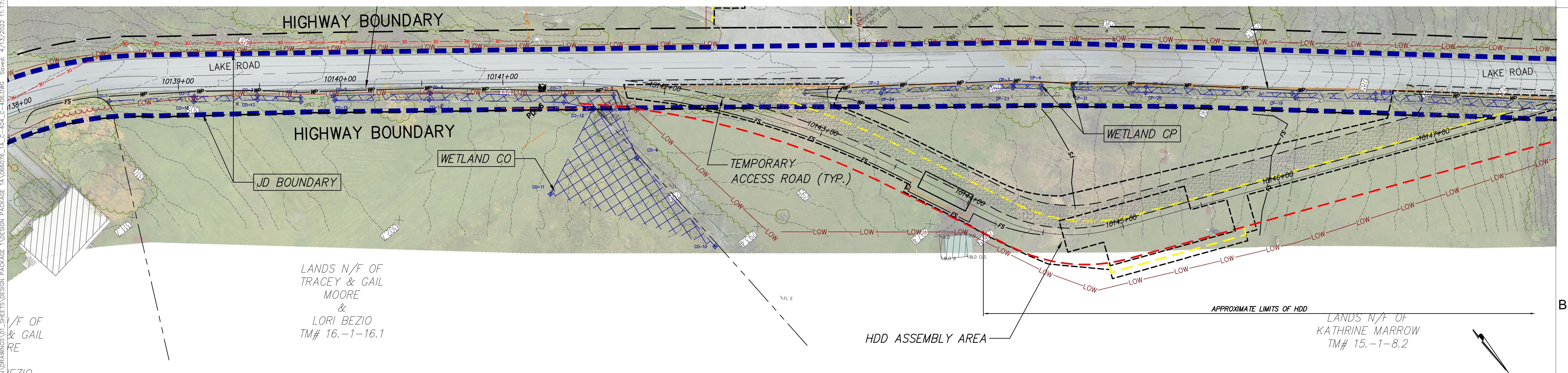
STA. 10135+00 TO STA. 10150+00 PLAN VIEW SCALE: 1" = 50'
